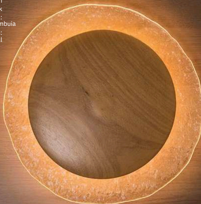
ARANDELA ECLIPSE PIASTRA GRANDE REF: 3451 Diâmetro: 0,45m Afastamento: 0,05m Fita LED 10,4W bivolt Fluxo luminoso: 1185 lm Temperatura de cor: 3000k Acabamento da madeira: BR Branco / PT Preto / CT Castanho / IB Imbuia Acabamento do vidro: 89 Ambar / 94 Cristal
