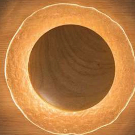
ARANDELA ECLIPSE PIASTRA PEQUENA REF: 3449 Diâmetro: 0,30m Afastamento: 0,05m Fita LED 6,6W bivolt Fluxo luminoso: 730lm Temperatura de cor: 3000k Acabamento da madeira: BR Branco / PT Preto / CT Castanho / IB Imbuia Acabamento do vidro: 89 Ambar / 94 Cristal
